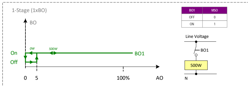
Fig. 26. Free Output: 1-Stage 1xBO
