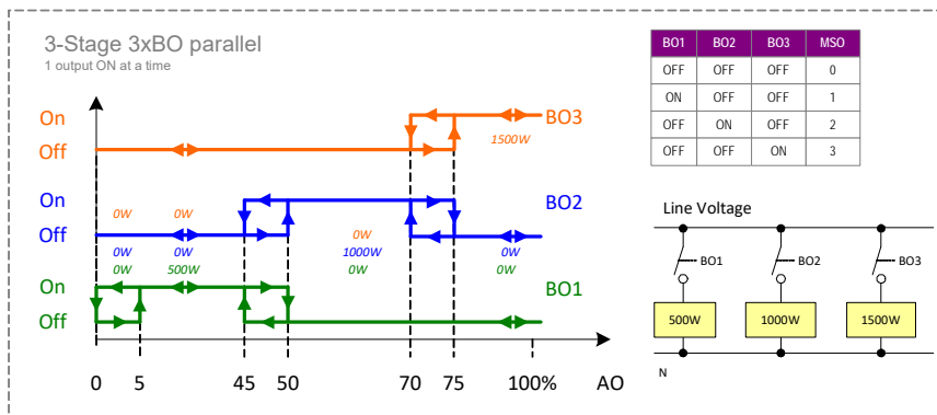
Fig. 30. Free Output: 3-Stage 3xBO parallel
