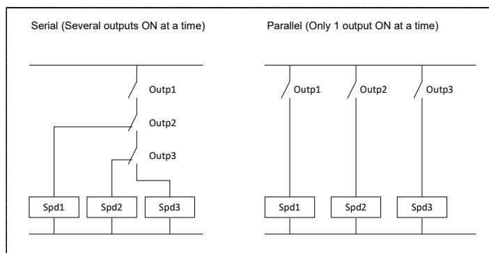
Fig. 19. Multi-speed fan wiring
