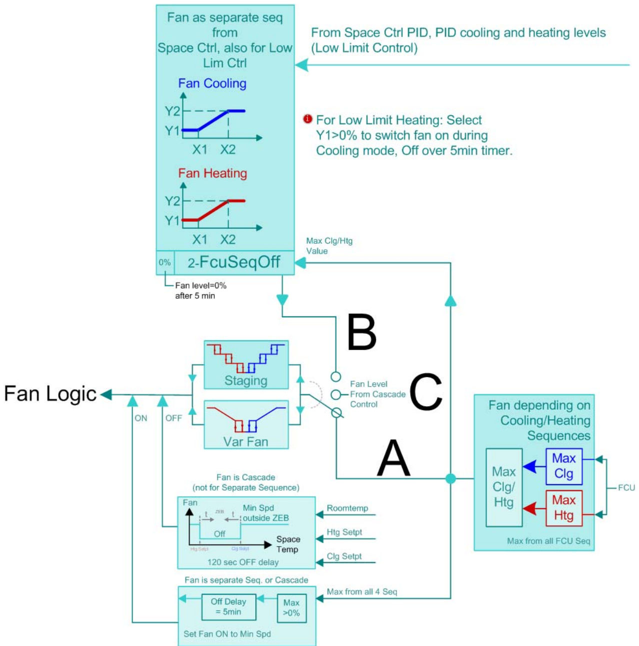
Fig. 23. Fan Control Strategy
