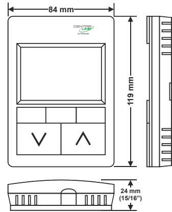
Fig. 2. LYNX wall module dimensions
