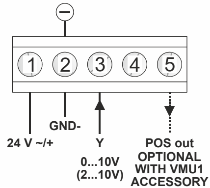
Fig. 9. Wiring
