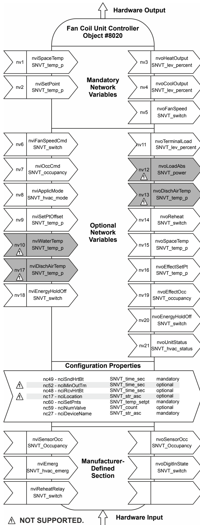
Fig. 7. LONMARK Fan Coil Unit object profile.
