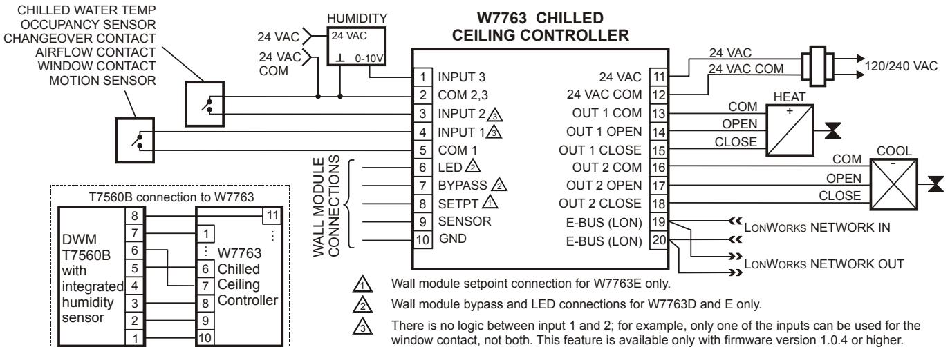
Fig. 4. Input/output details
